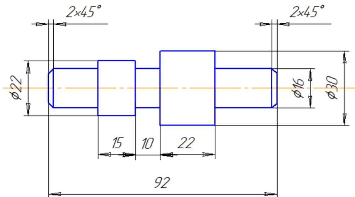
Рис. 1. Чертеж «Вал»
